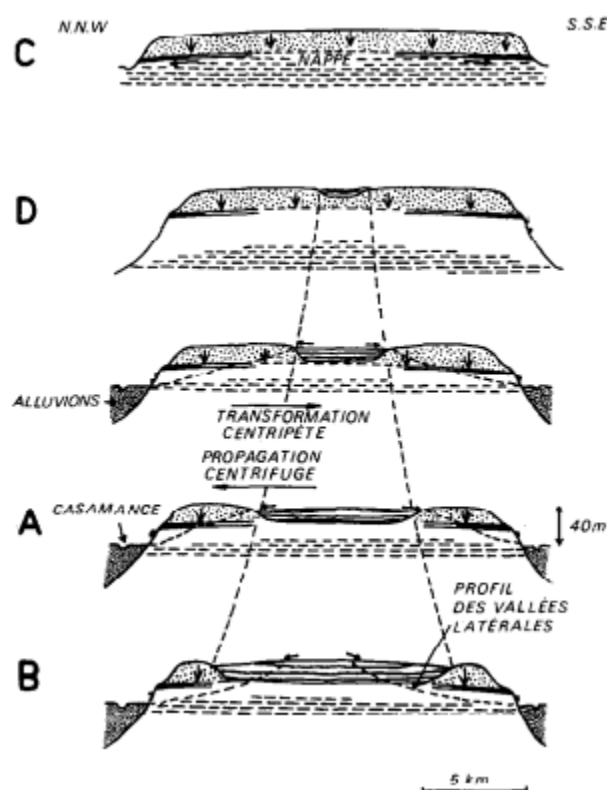
FIG. 10 - Étapes successives supposées de l'évolution d'un plateau de moyenne Casamance (C, D, A, B).
